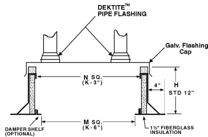
Dektite Pipe Curb DPC RF
